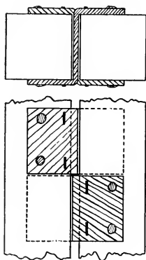
Fig. 259—Leather Hinge
